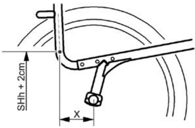
Achterwielpositie
